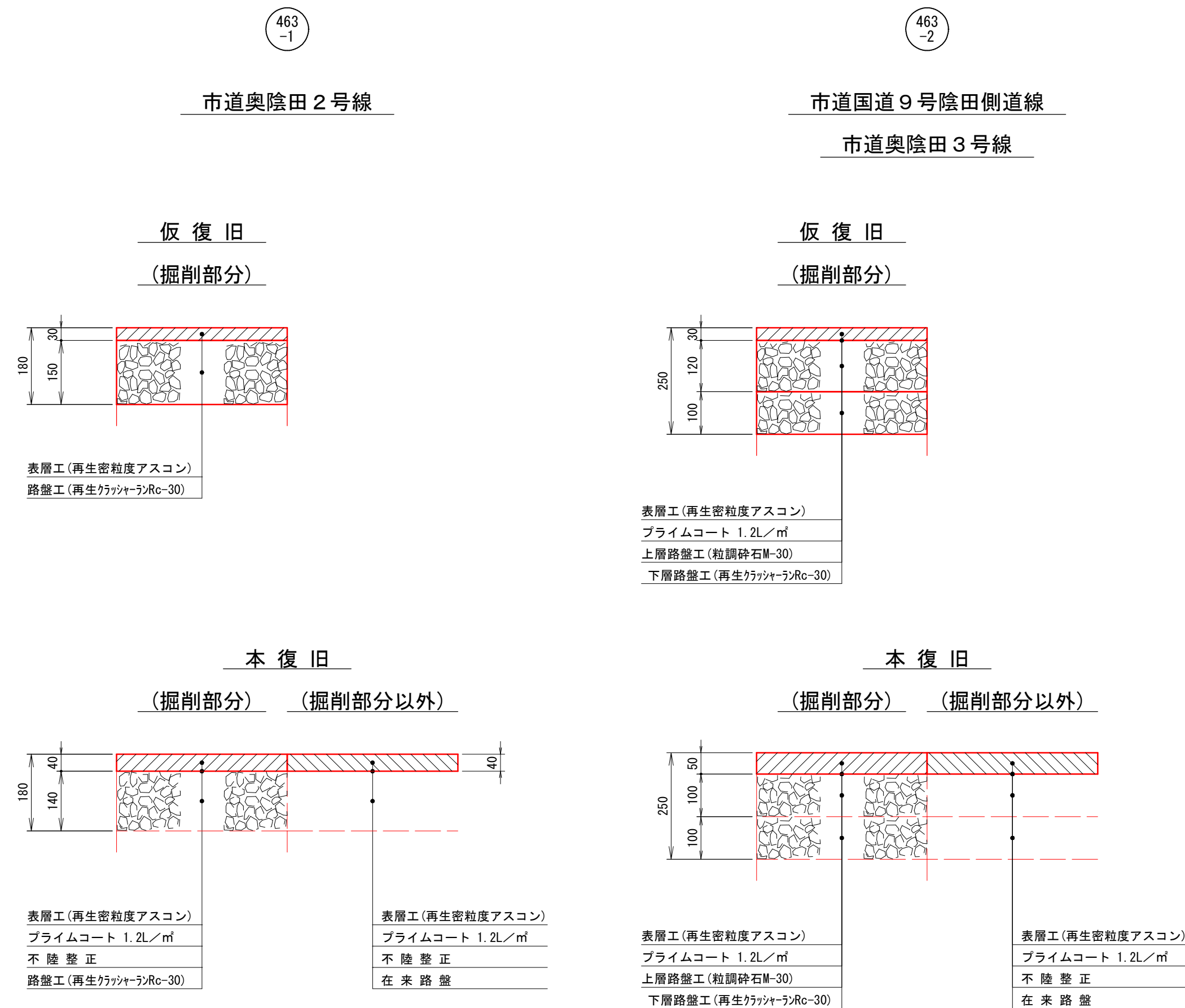
舗装復旧断面図 縮 尺 1:10
