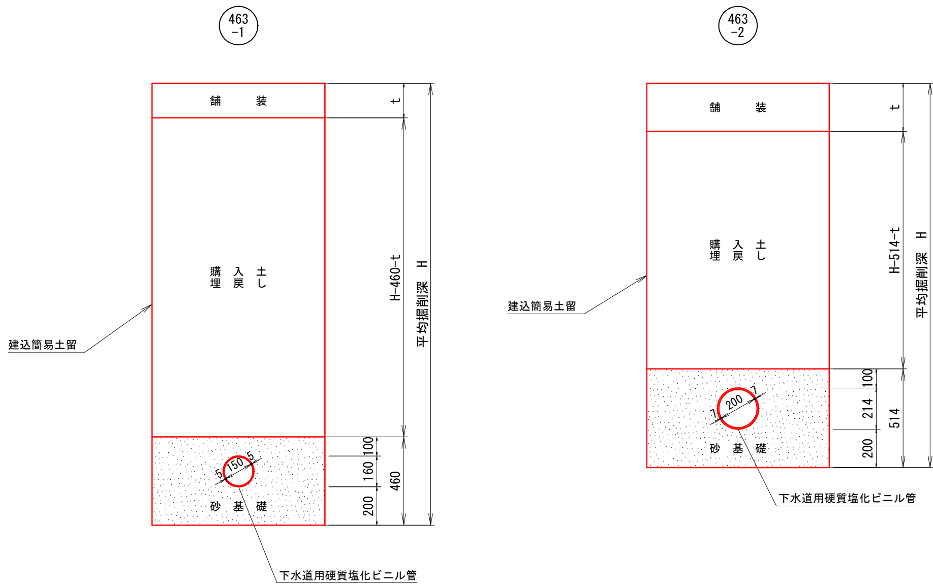
掘削標準断面図
