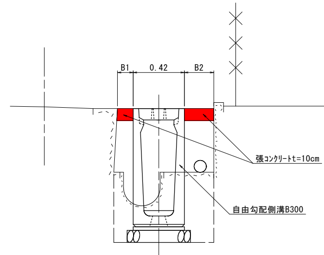
張コンクリート S=1:20
