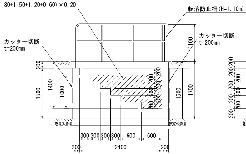
側面図
