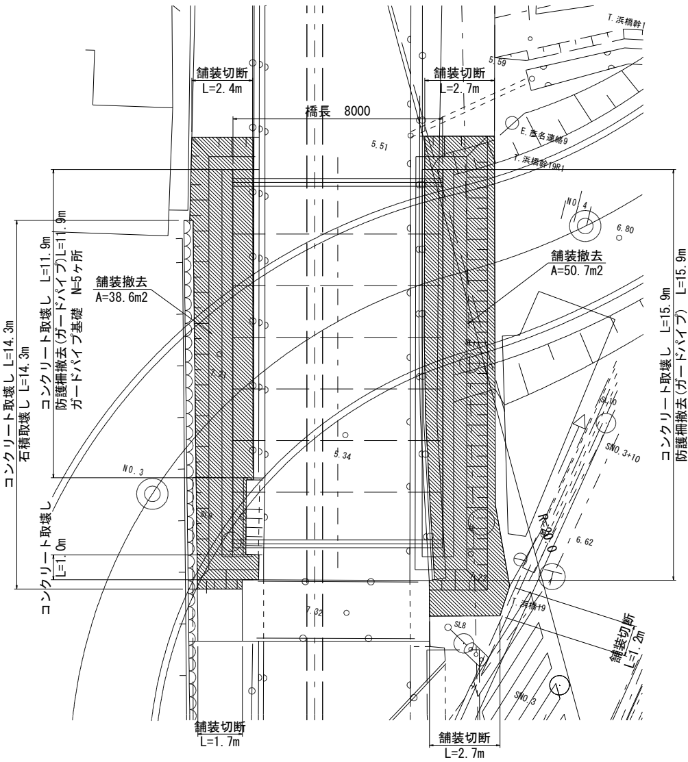
平面図
