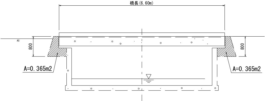
歩道橋平面図
