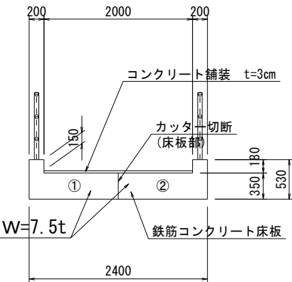
歩道橋断面図
