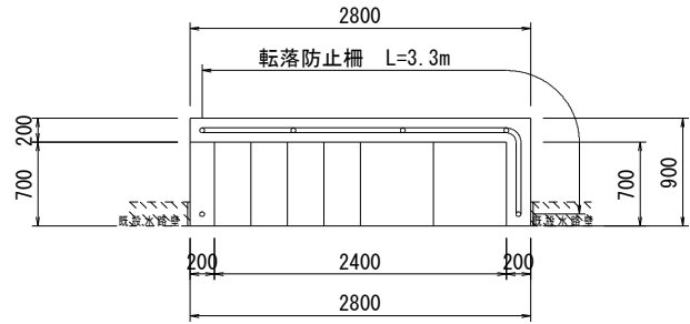
側面図
