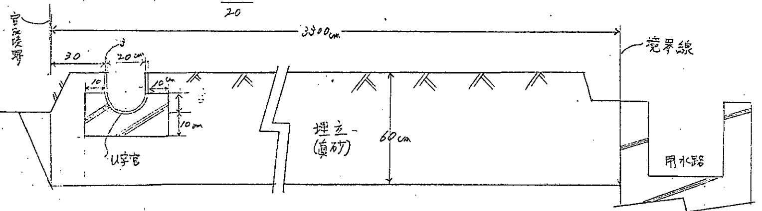
B~B'断面図
