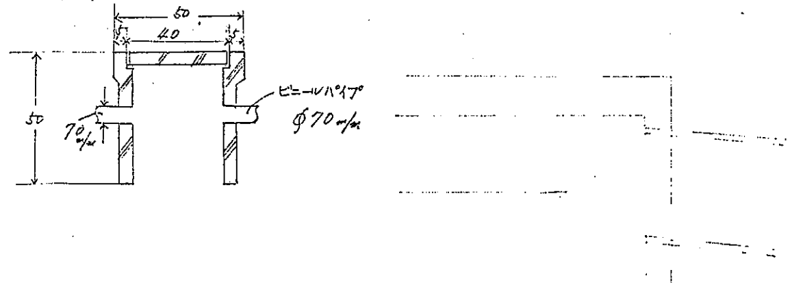
溜折断面図 (2次製品 400×400×500)
