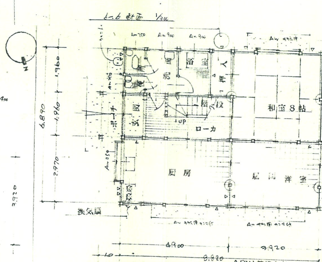
1階平面図 1:100
