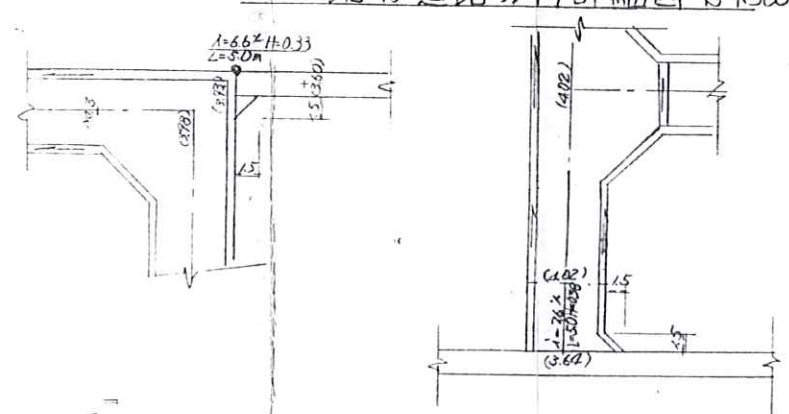
既存道路取付詳細図 S=1:500
