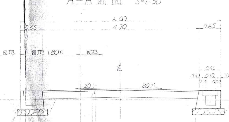
A-A断面 S=1:50
