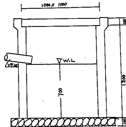
現況断面図
