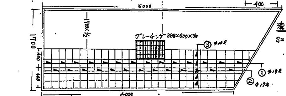
コンクリート擁壁 S = 1 / 20
