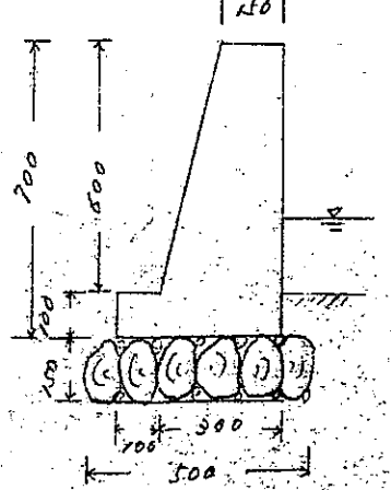
擁壁の詳細図
