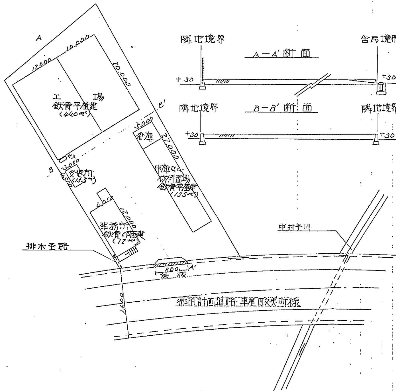
敷地現況図 1/500
