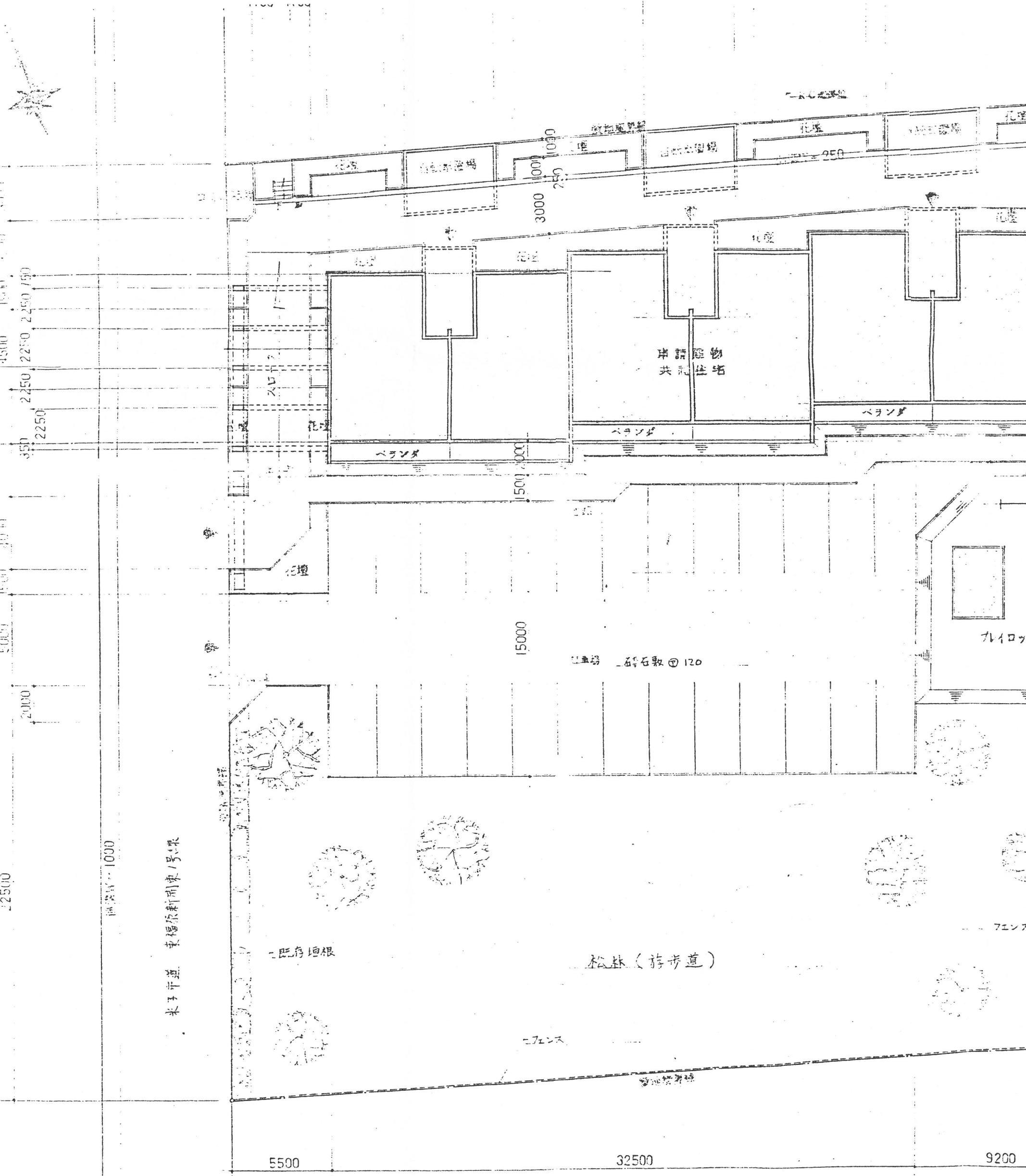
敷地配置図 5+1:200
