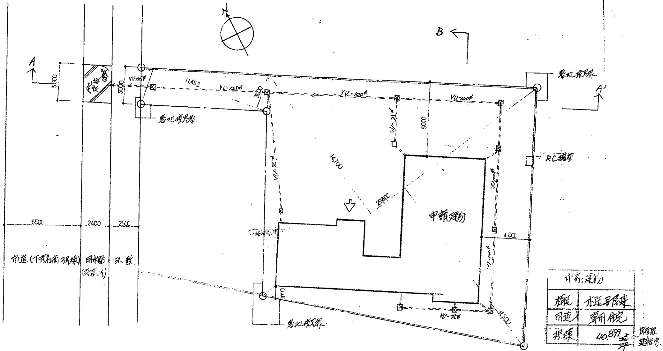
配置図 1/200
