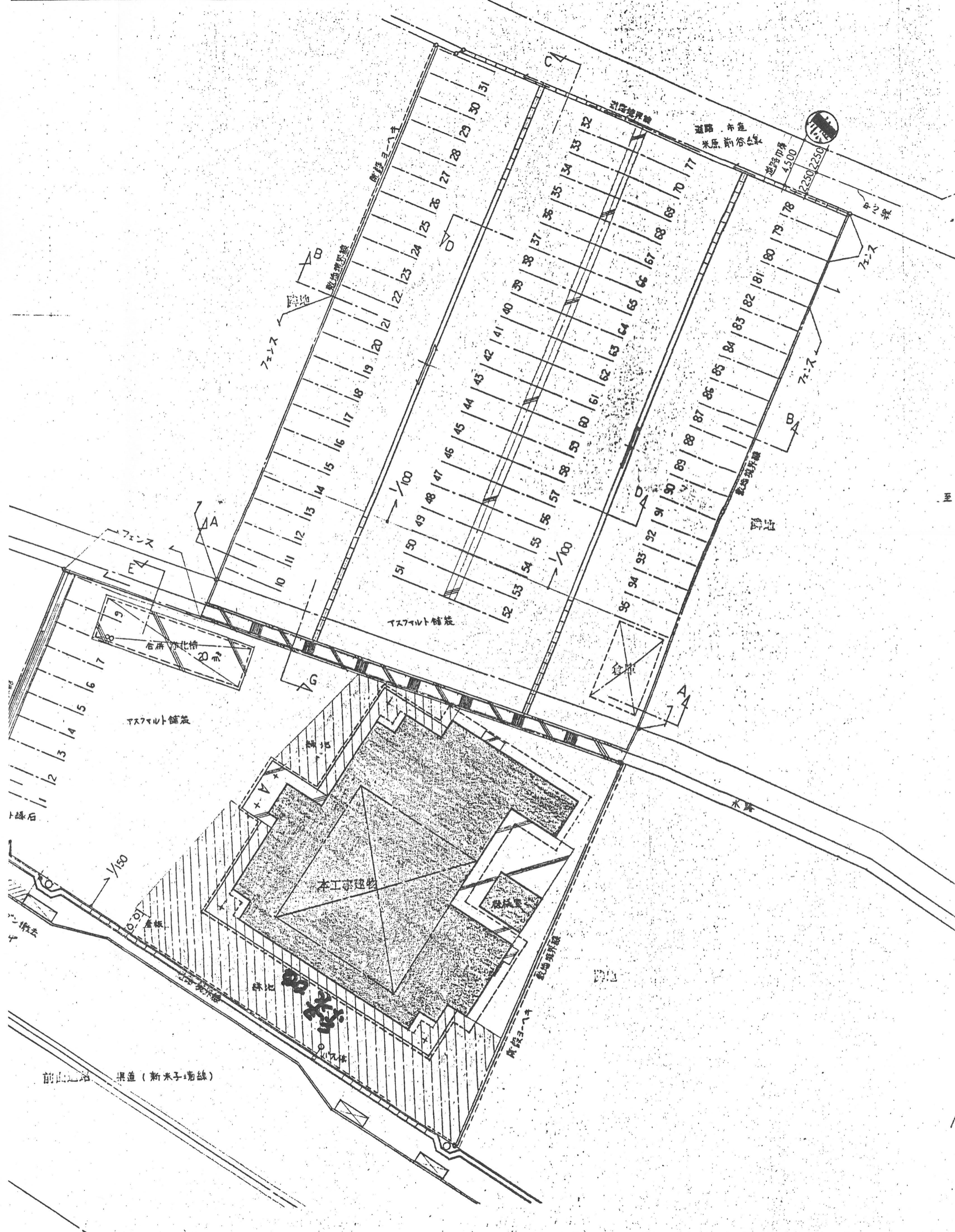
配置図 | S-1/600
