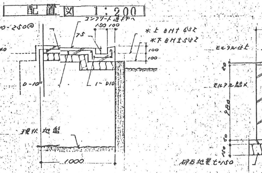
C~C 断面図 1:30
