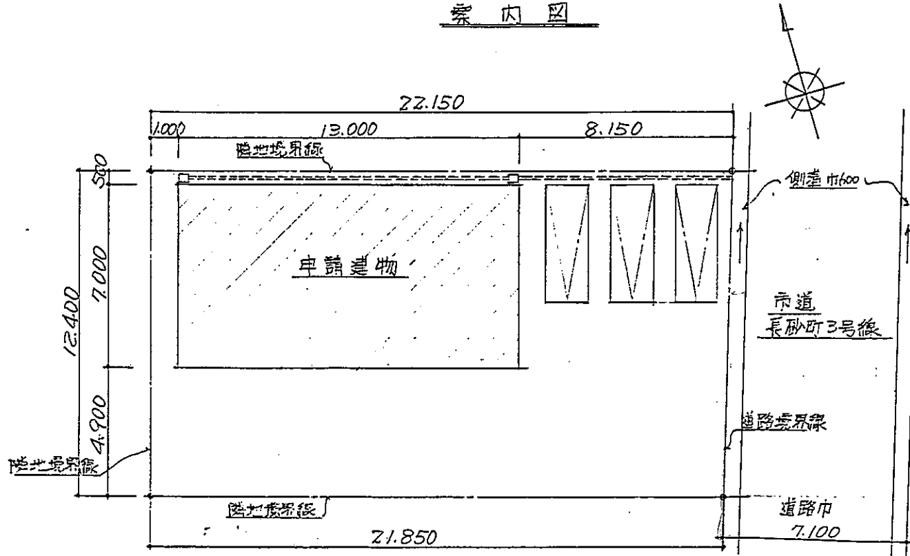
配置図 1/200
