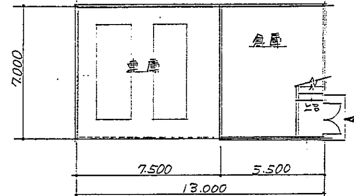
1階平面図 1/200
