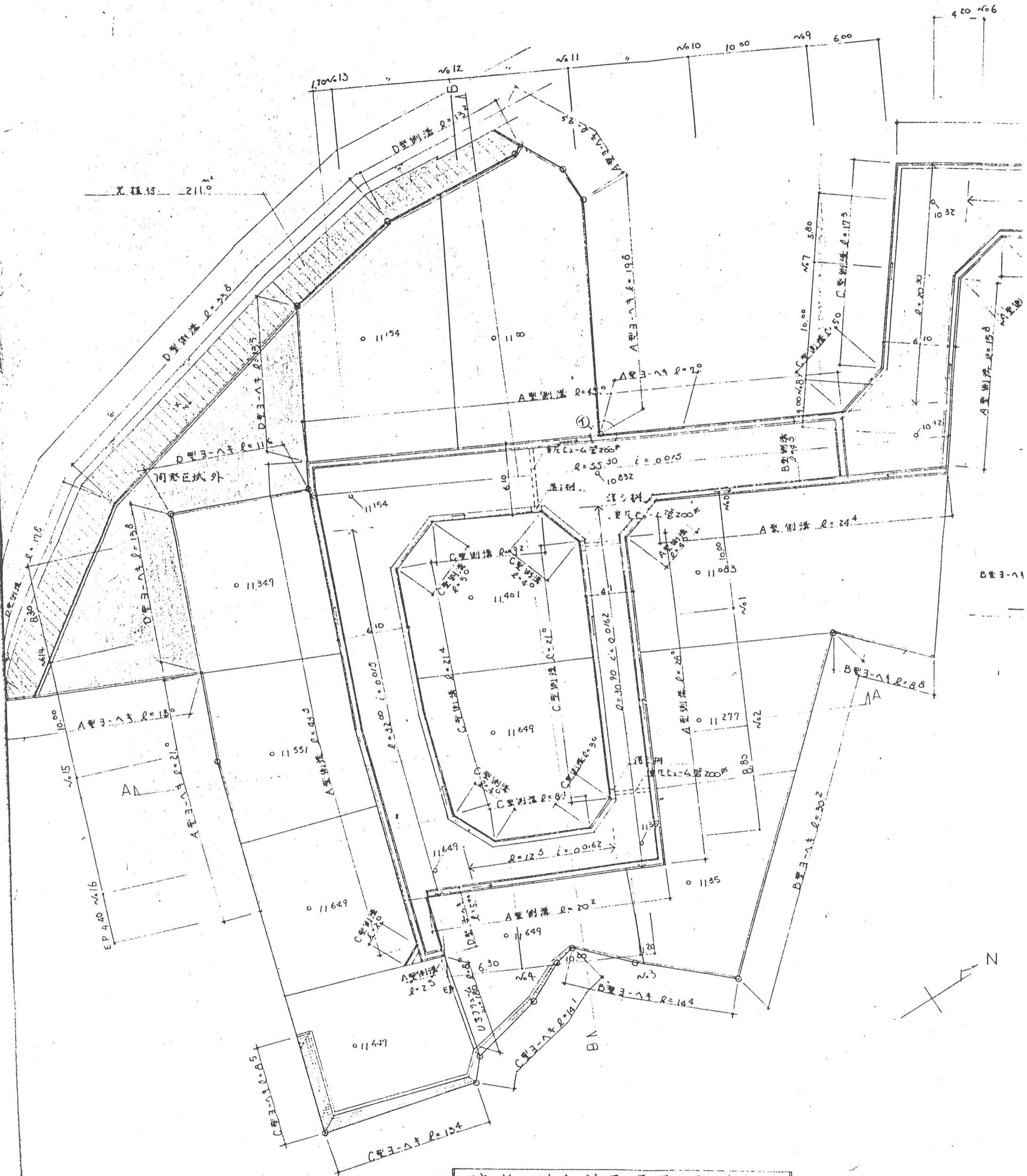
完成·排水計画平面図 1:300
