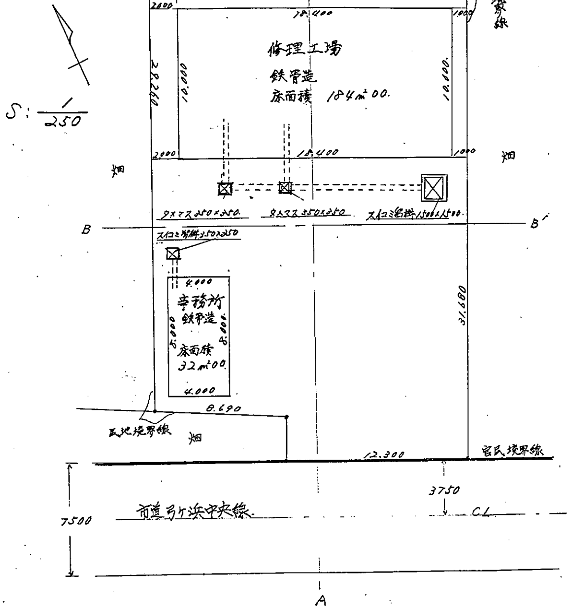
敷地現況図
