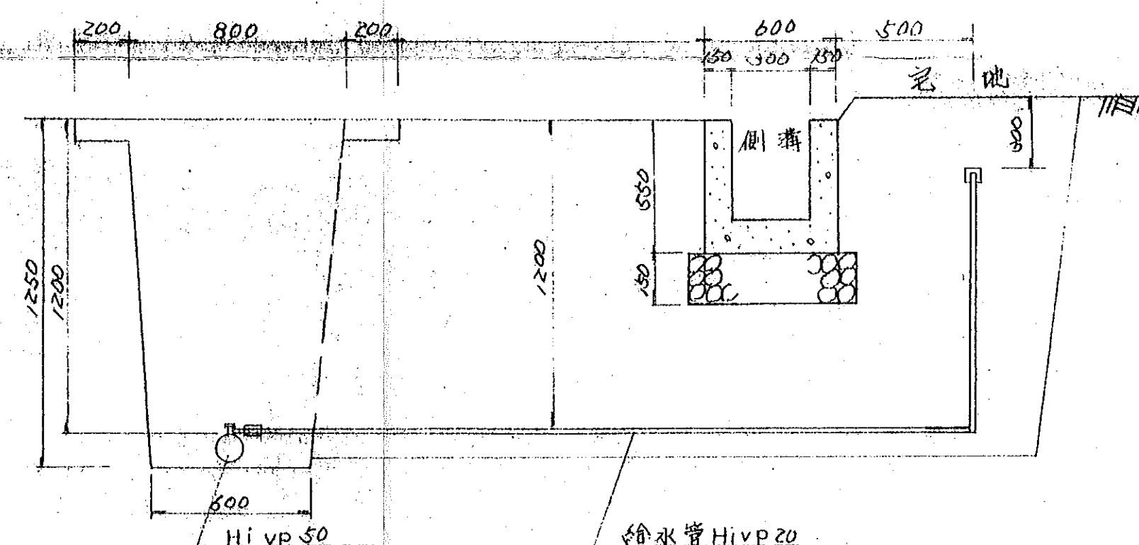
断面図
