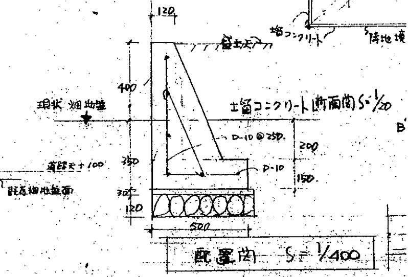
B~B' 断面図 S=1/300
