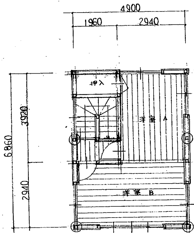
2F 平面図 S=1/100
