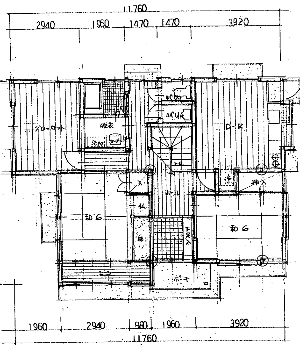
1F 平面図 S=1/100
