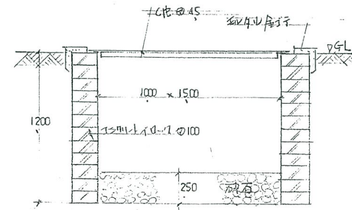
吸水研断面図
