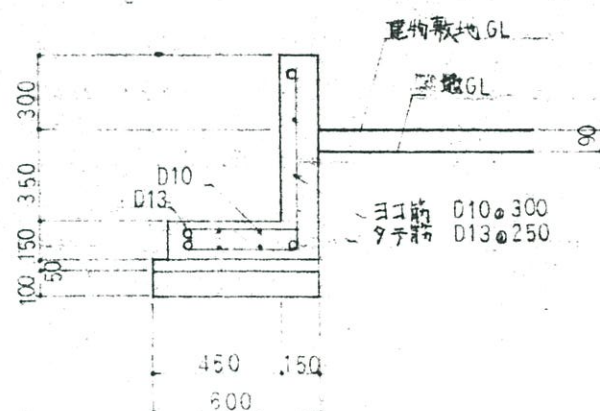
b 断面図 S=1:30
