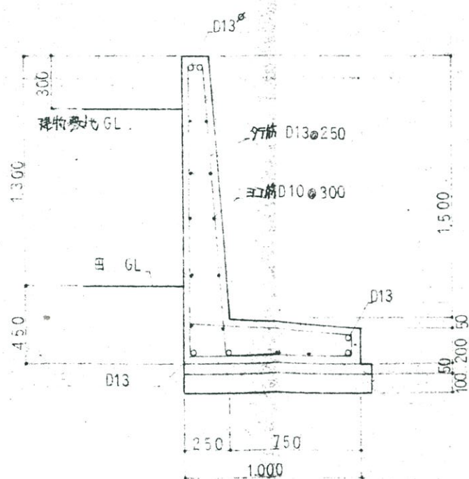
a 断面図 S=1:30
