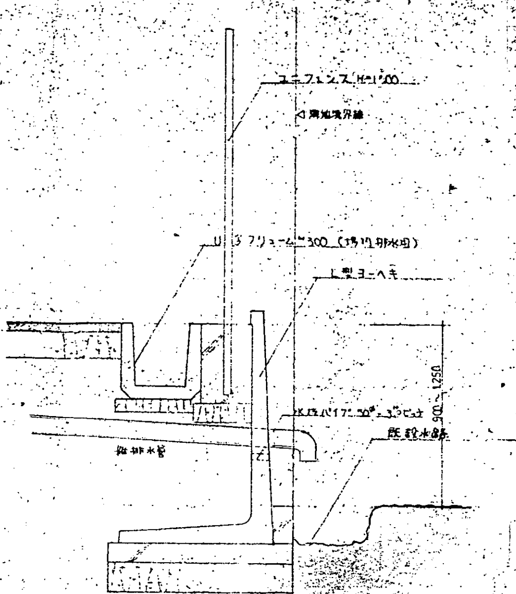
A-A 断面図 1/20
