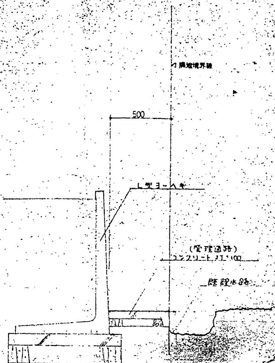
B-B 断面図 1/20
