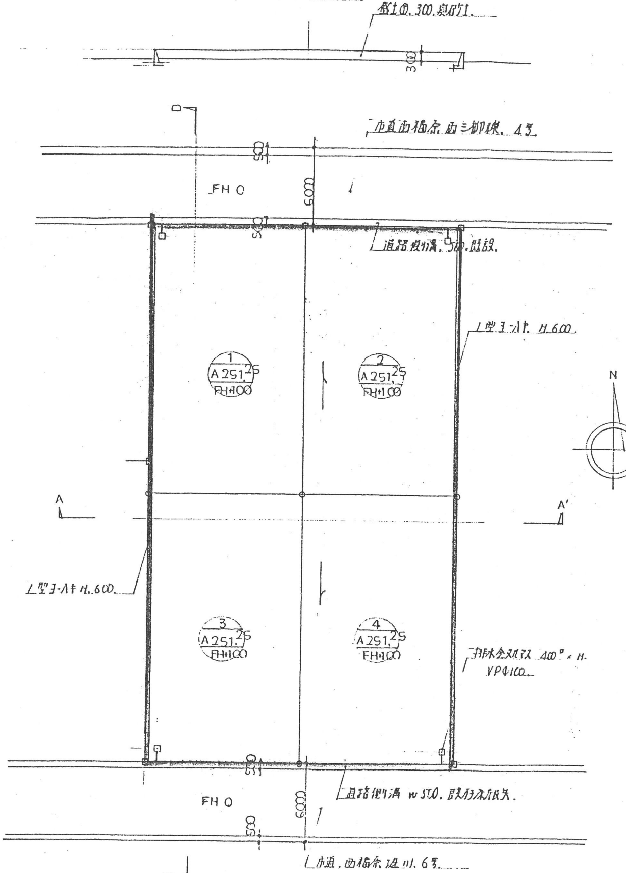
工池利用計画図，遊具計画平面図。1:300
