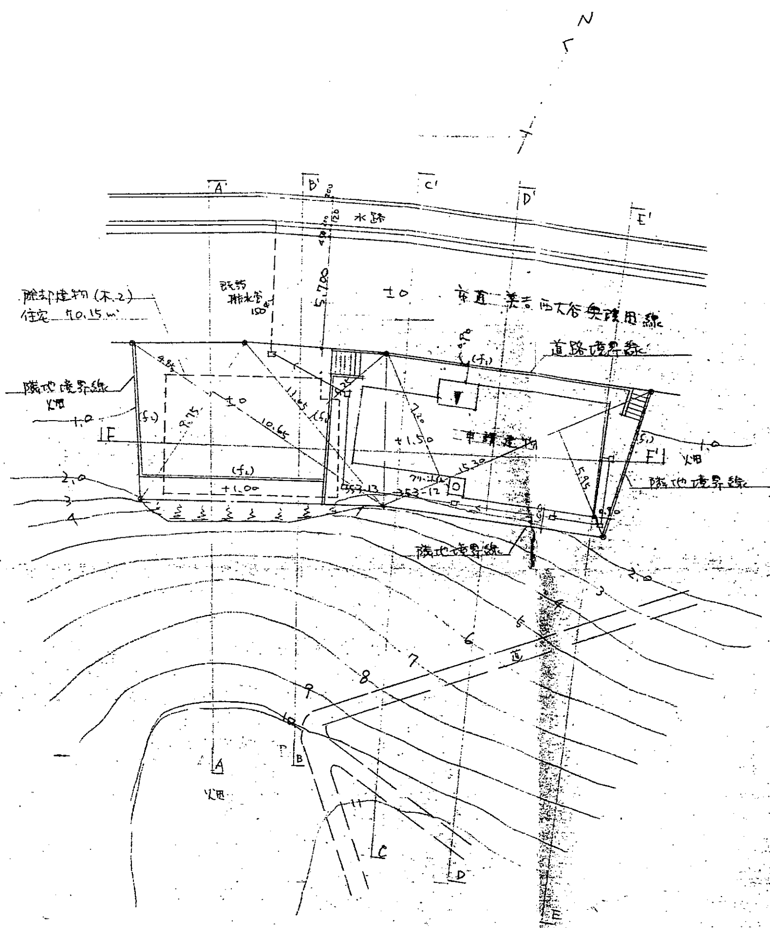
配置図 土地利用計画図 1/200
