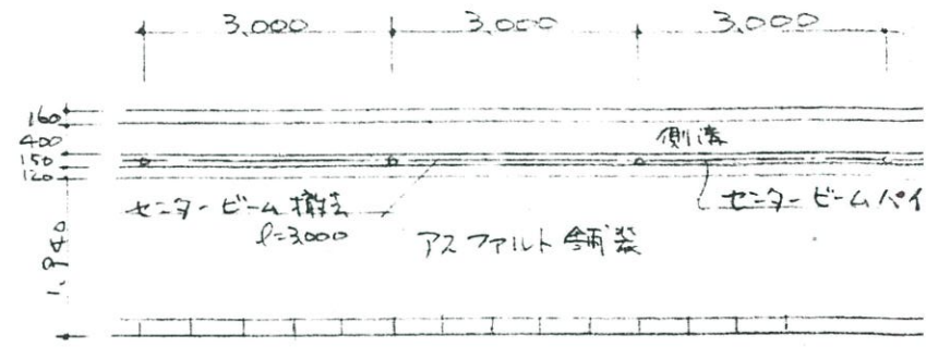
現況平面図 \frac{1}{100}
