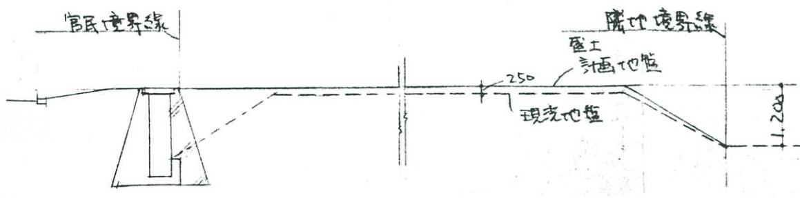
A~A' 計画断面 \frac{1}{100}
