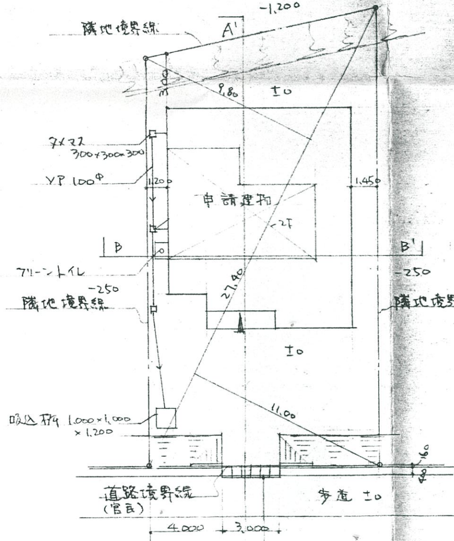
配置図 \frac{1}{200}
