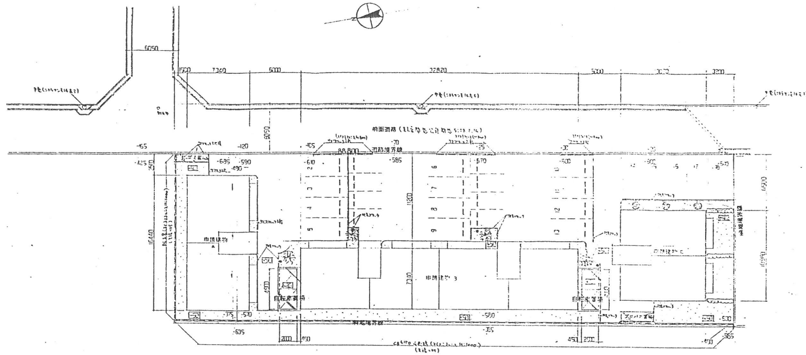
配 置 図 1/200
