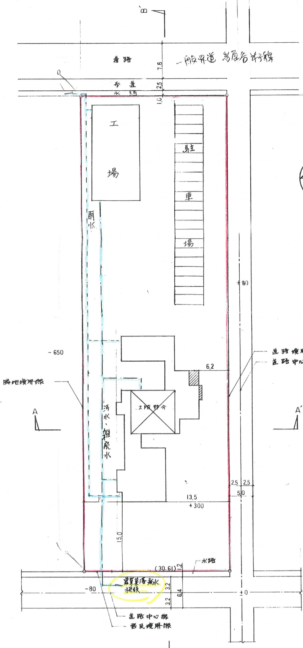
配置図 1/500
