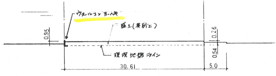
A - A' 断面図 1/500
