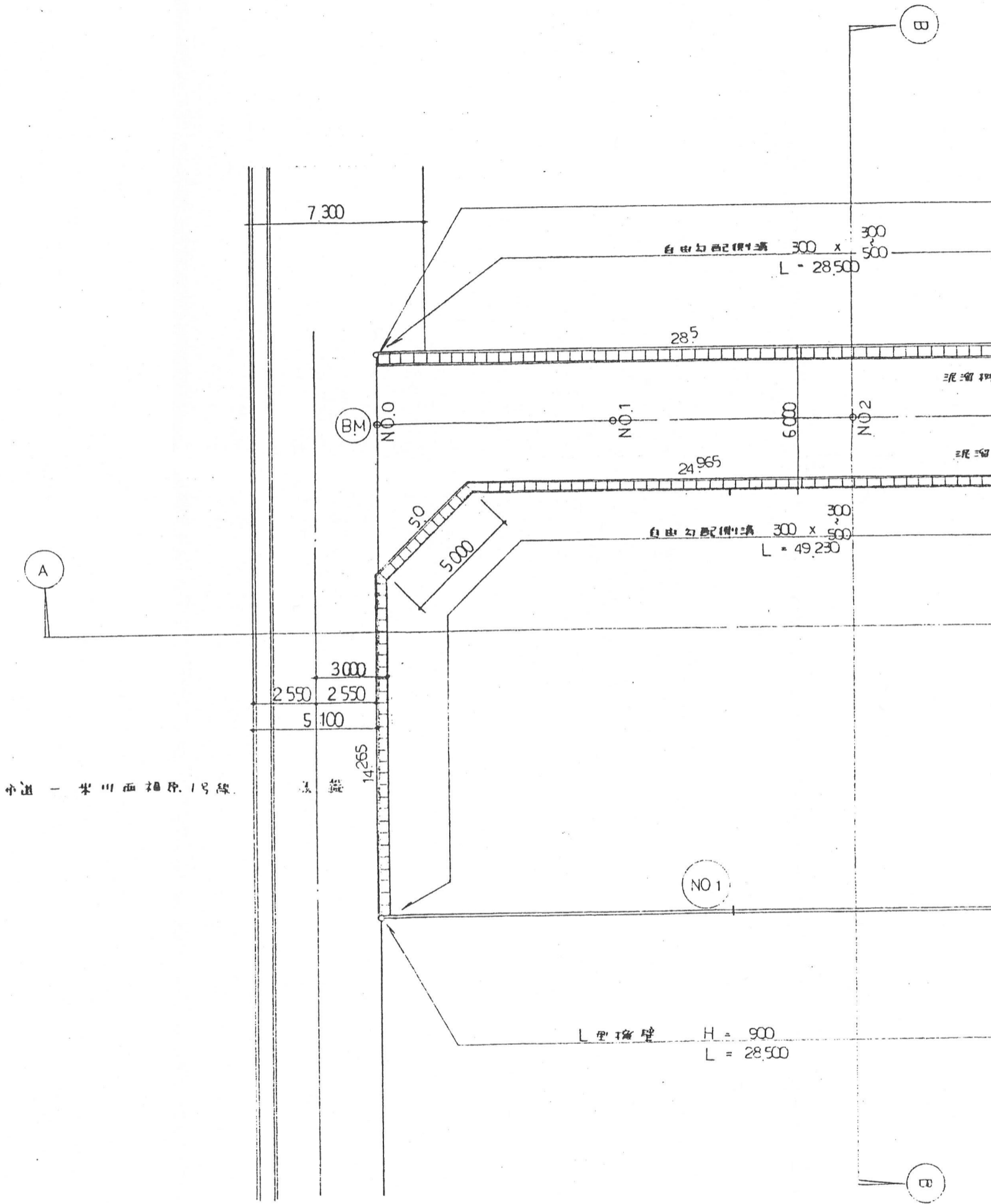
造成計画平面図
