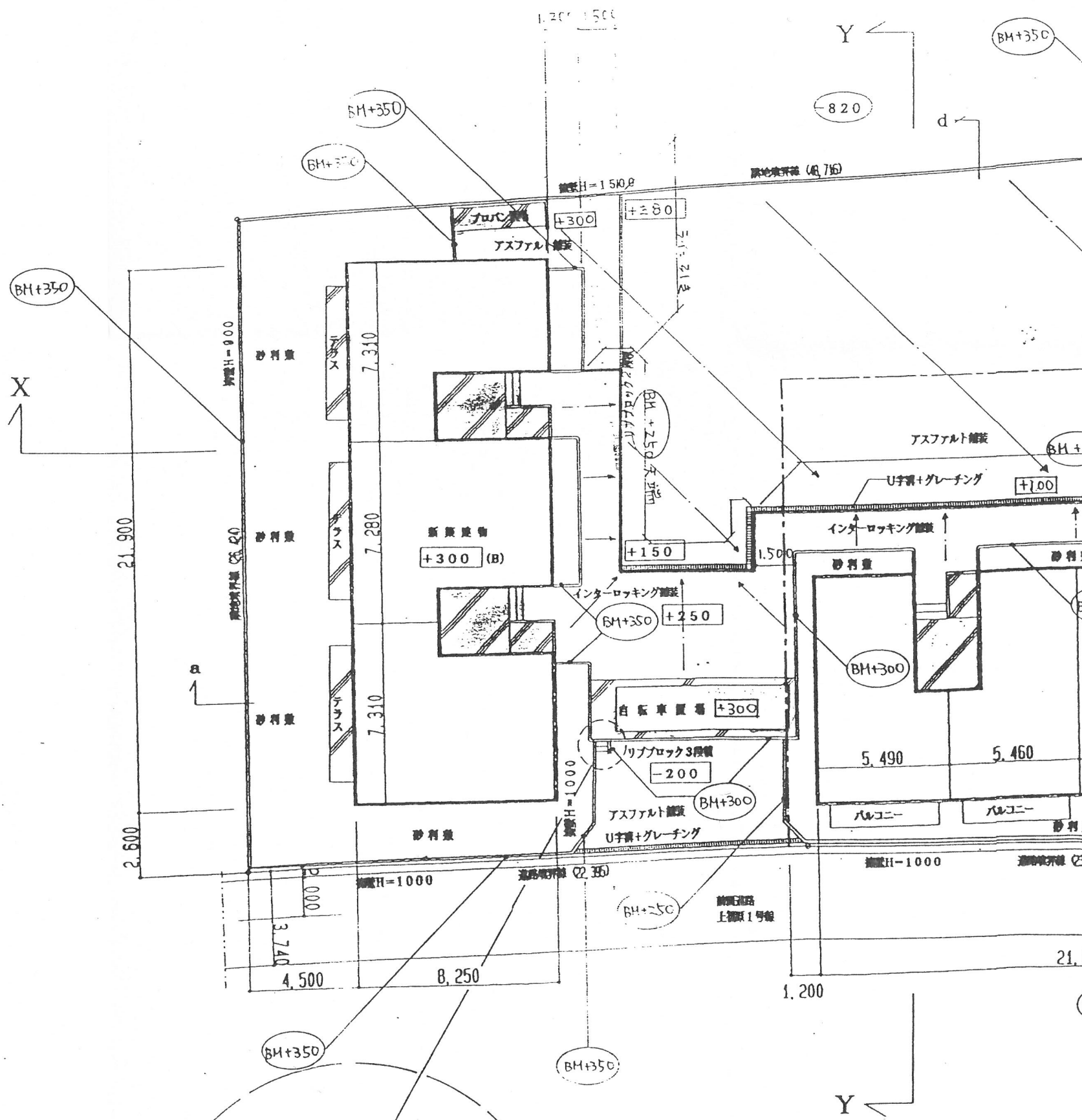
土地利用計画図 1 / 200
