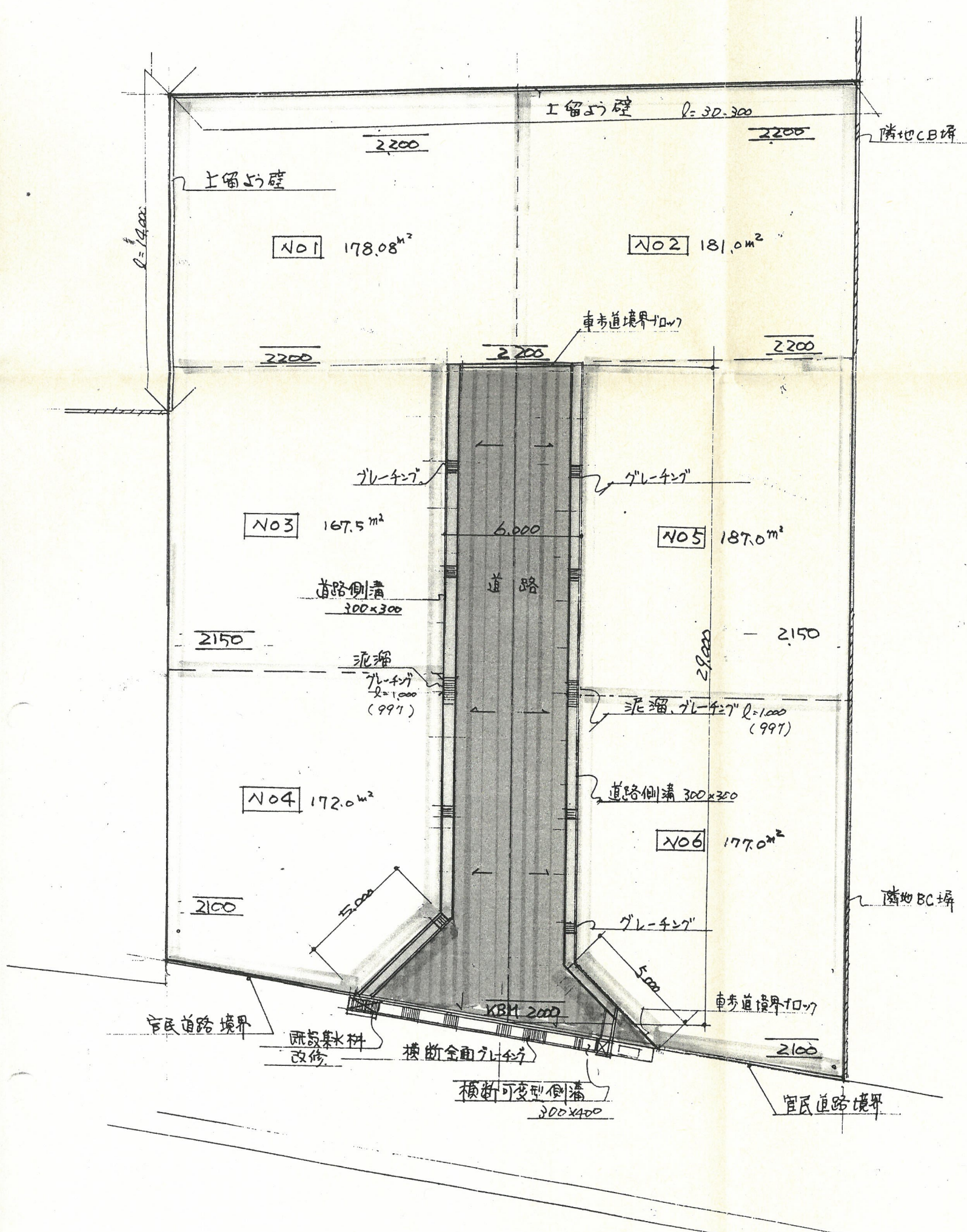
道路断面の側溝の配列図に示す
