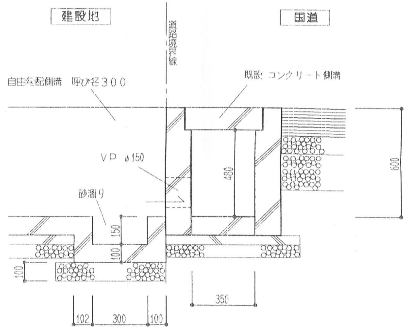
D-部 断面詳細図 S=1/20
