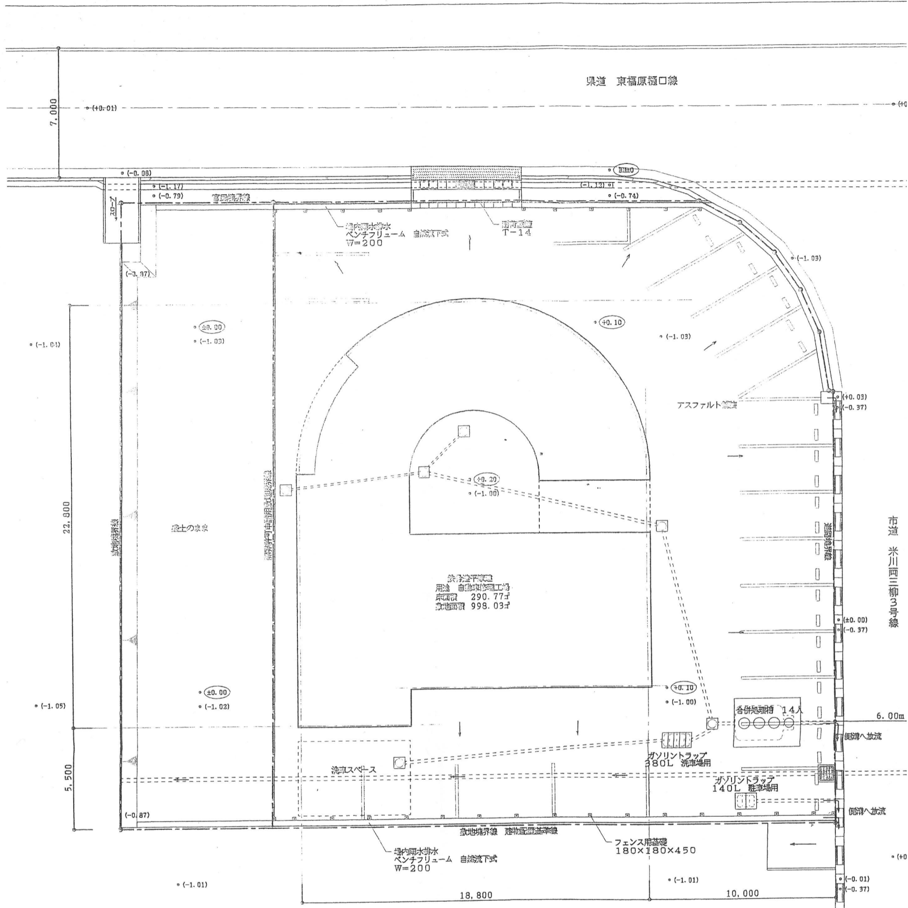
造成工事平面図 31:200
