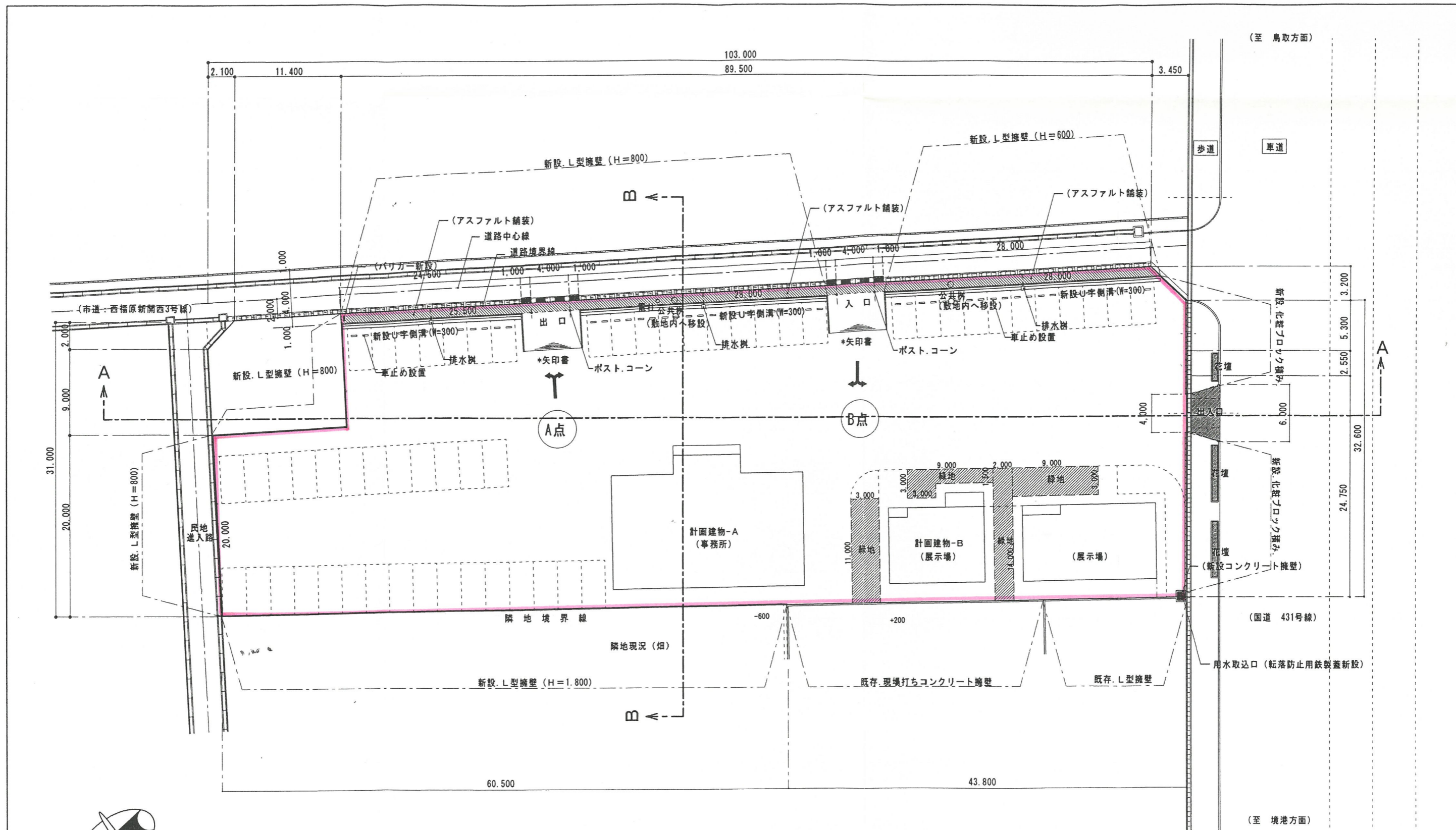
計画平面図 S=1:400
