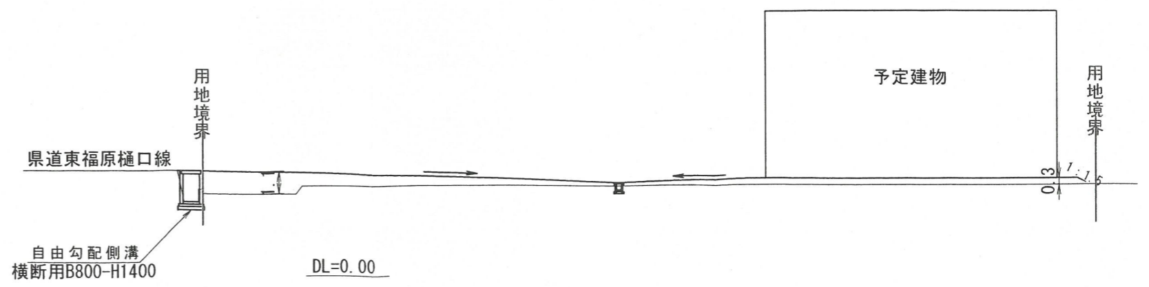
B-B' S=1:250
