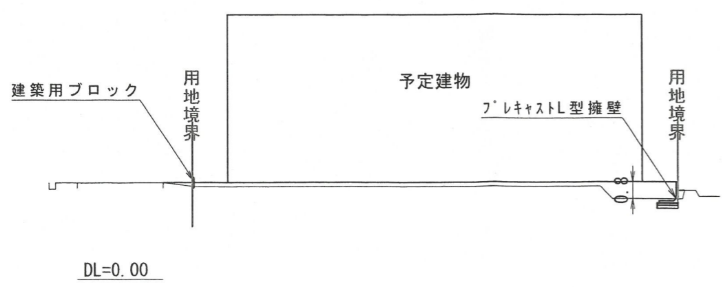
A-A' S=1:250
