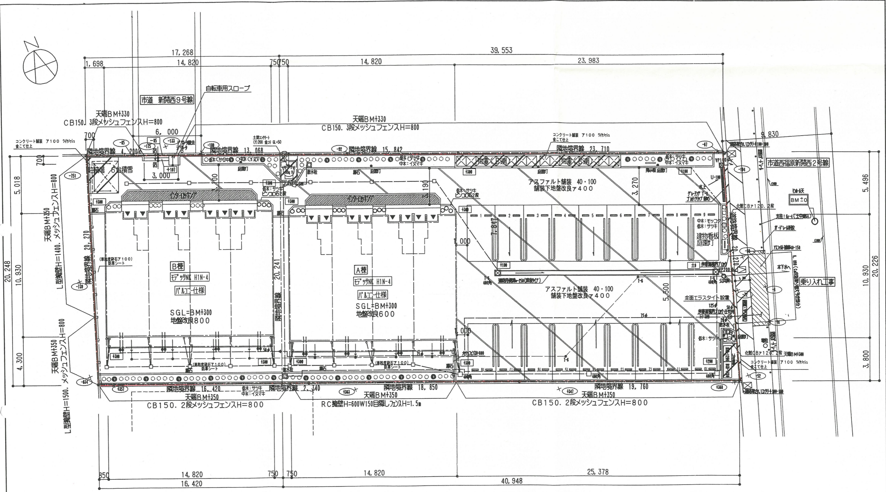
計画配置図 S=1:200
