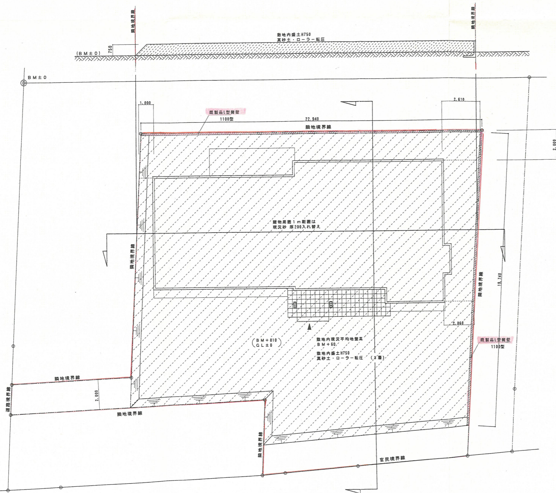
造成図 S. 1/150 敷地面積 490.12m 2
