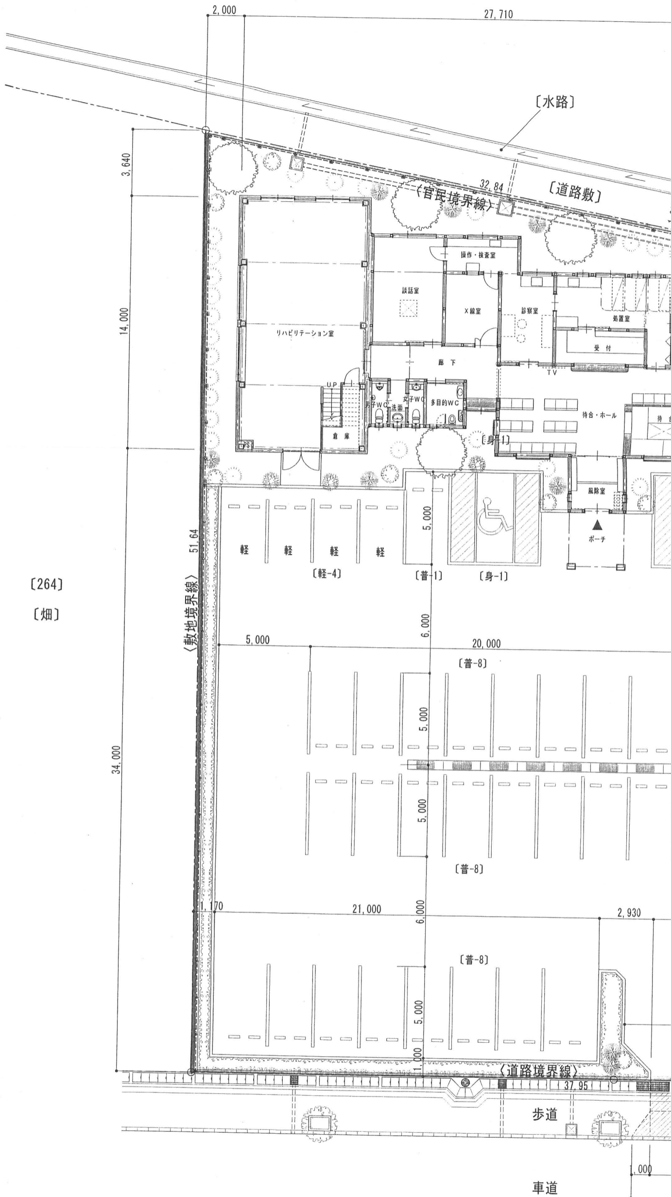
造成計画平面図.2 S=1:200
