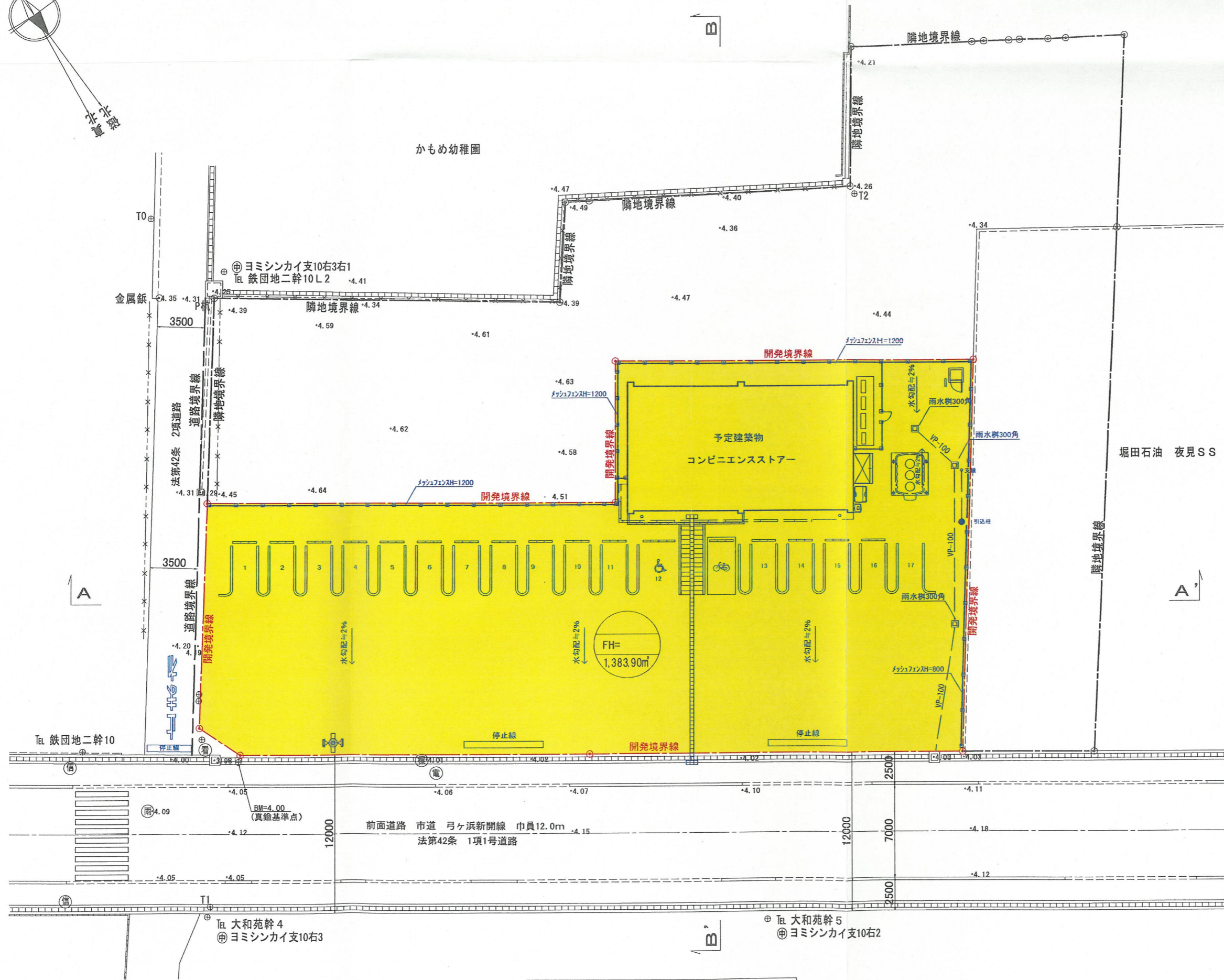
土地利用計画平面図 S=1:300
