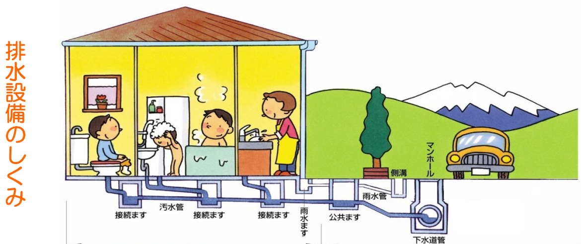
排水設備（個人が設置・管理する部分） 公共下水道（米子市が設置・管理する部分）
