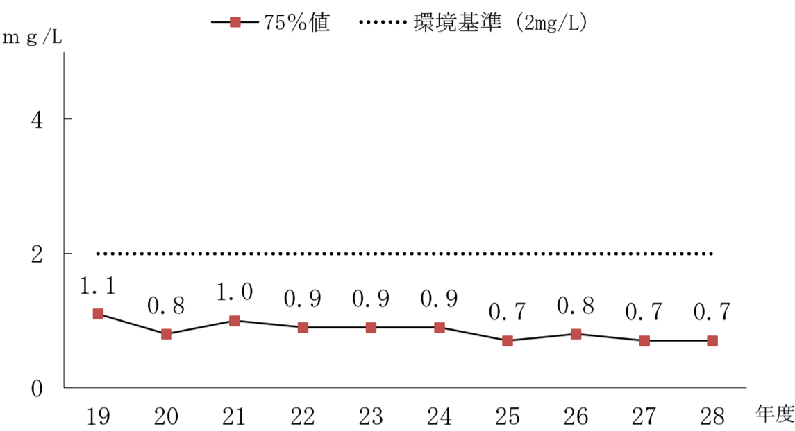
日野川（皆生）
