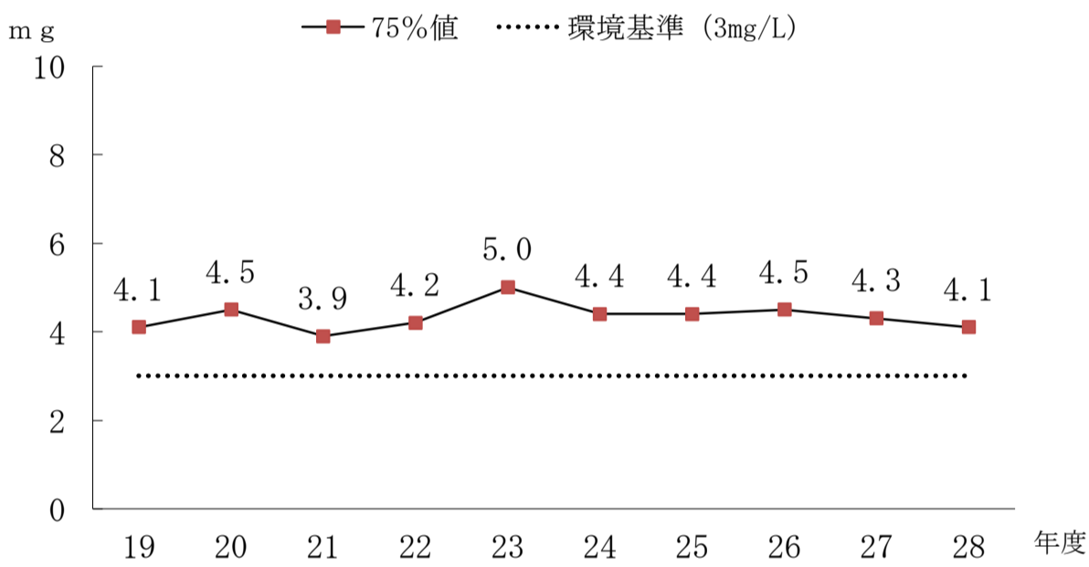
彦名町地先
