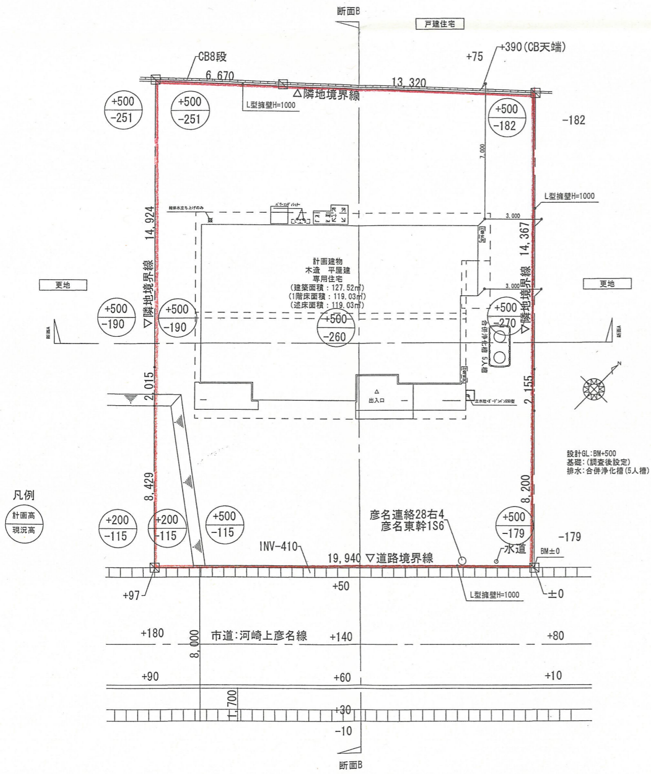
配置図 S:1/200
