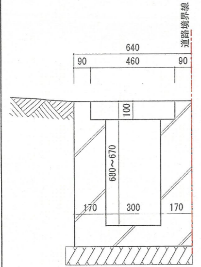
道路側溝断面図 1:20
