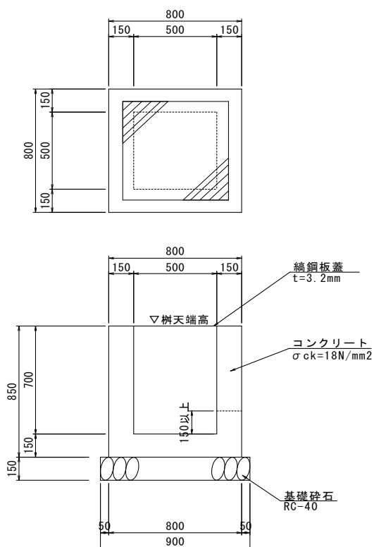
2号集水桧 (B500-L500-H700) 流入・流出概略図
