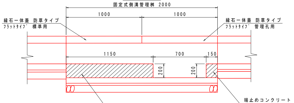
側 面 図
