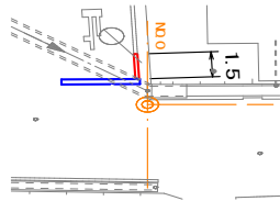
平面図 S=1:300 NO. 0付近
