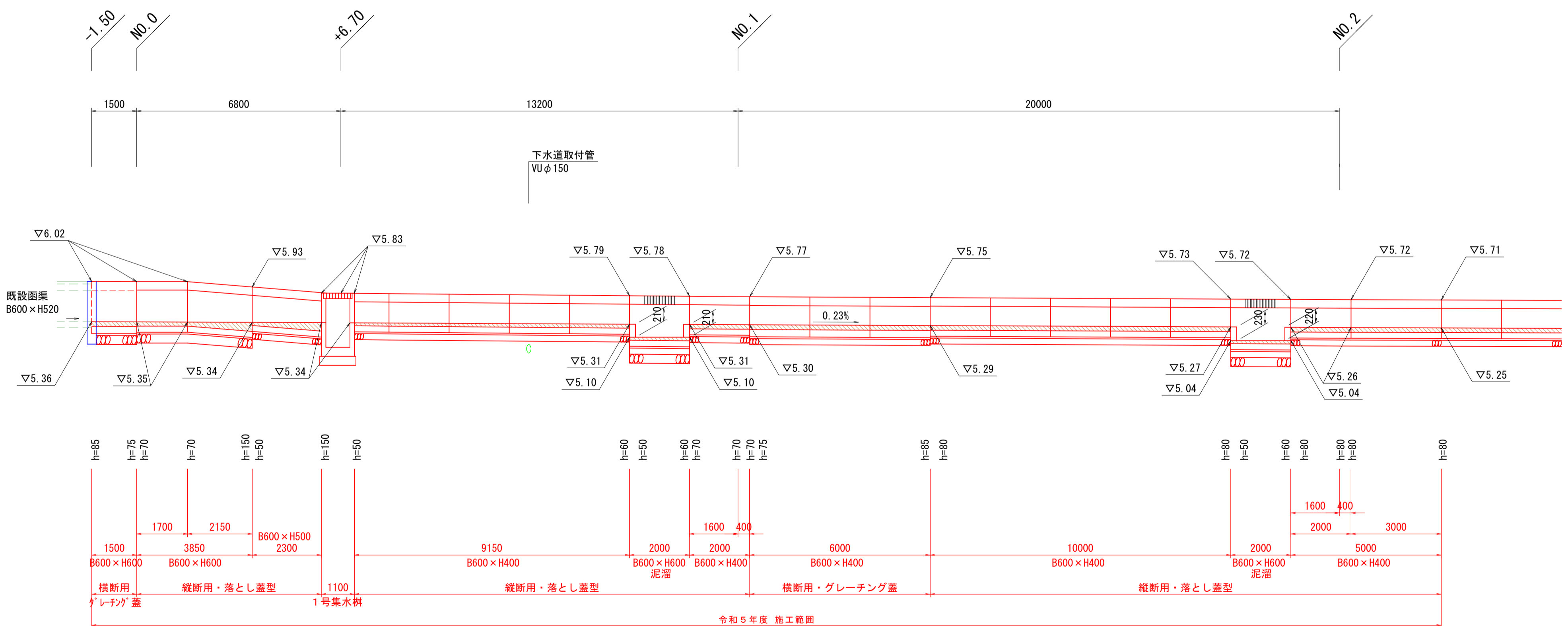
展開図 H=1:100 V=1:50
