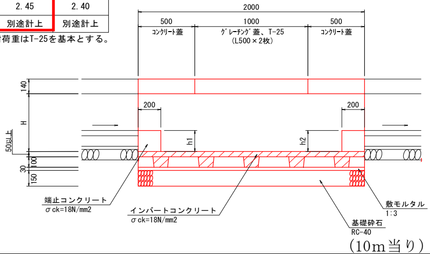
側面図
