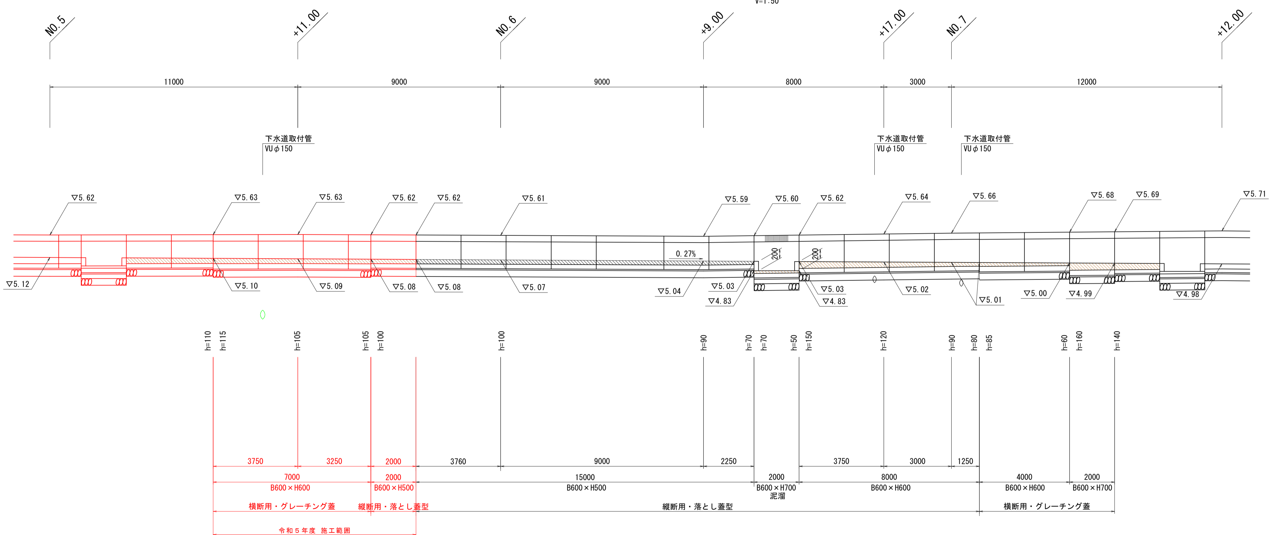
展開図 H=1:100 V=1:50
