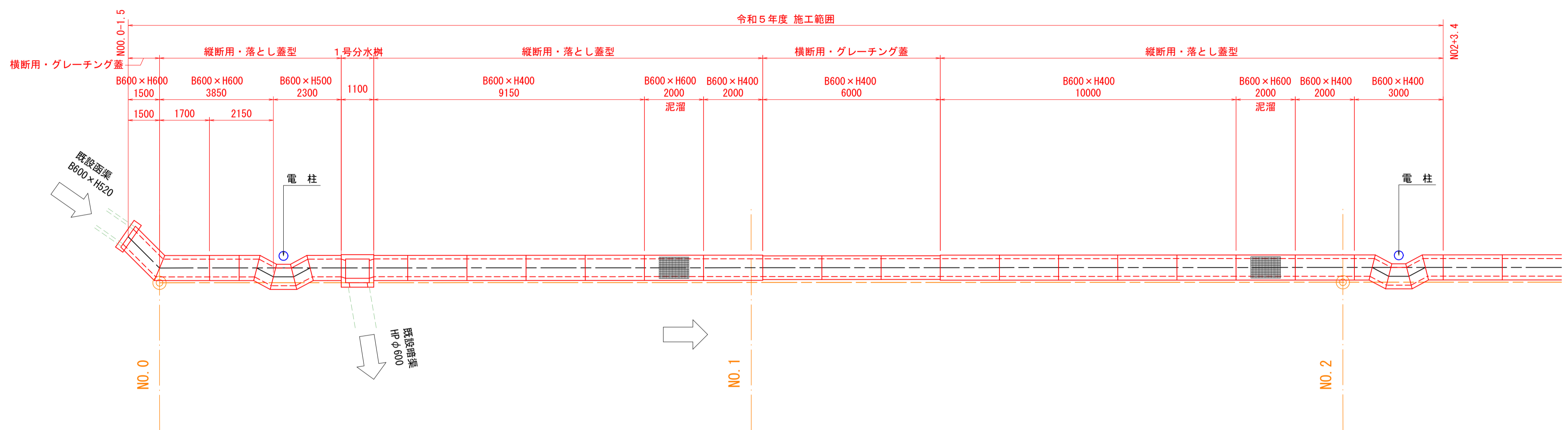
展開図 H=1:100 V=1:50
