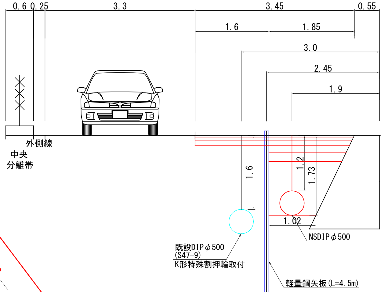
断面図 S=1:50
