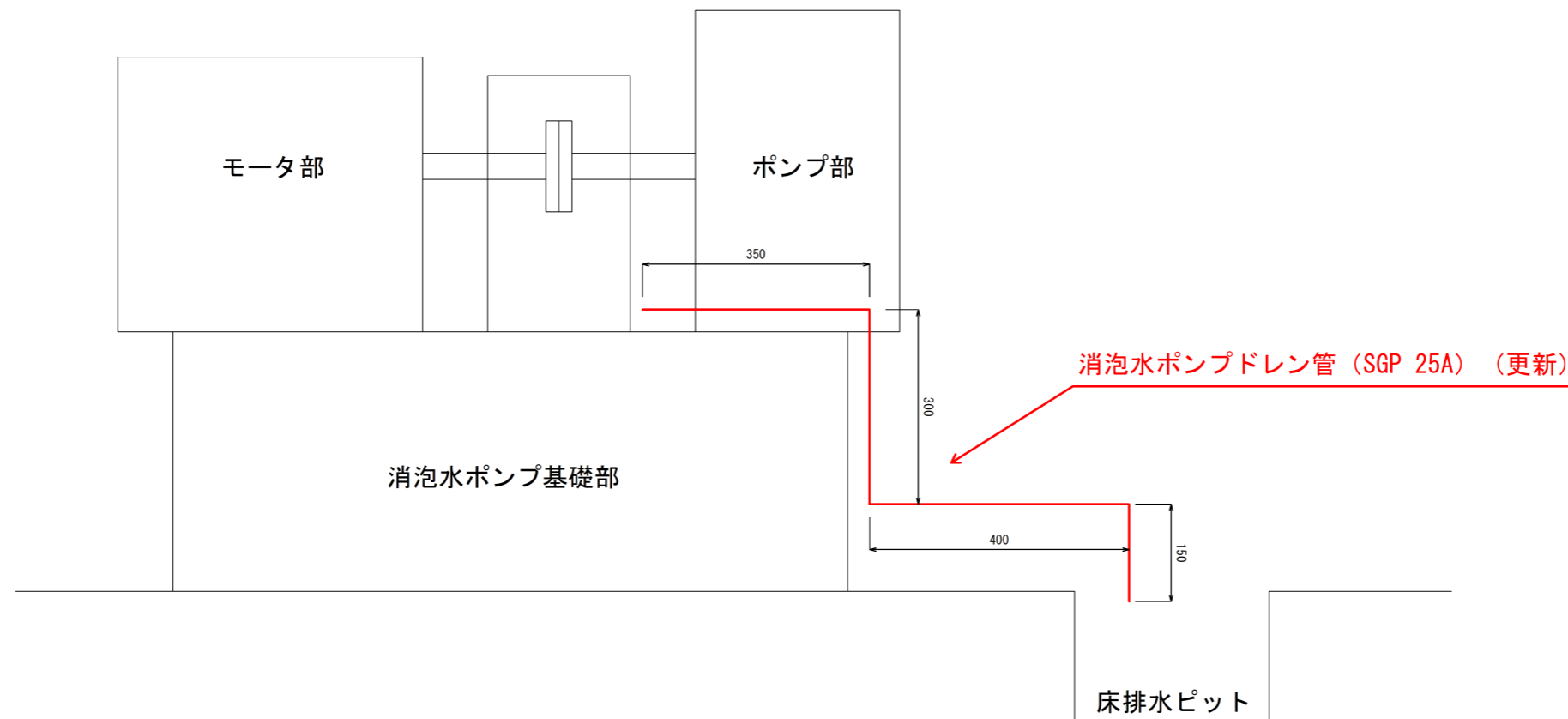
消泡水ポンプドレン管詳細図
