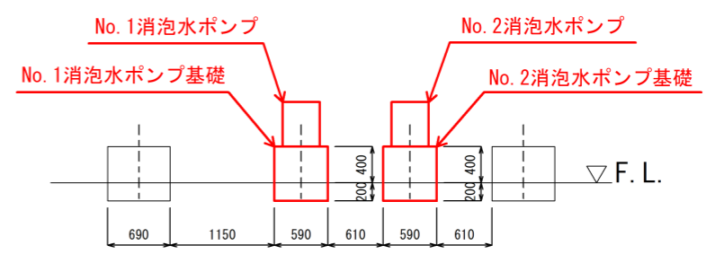
A-A断面図 (S=1/75)
