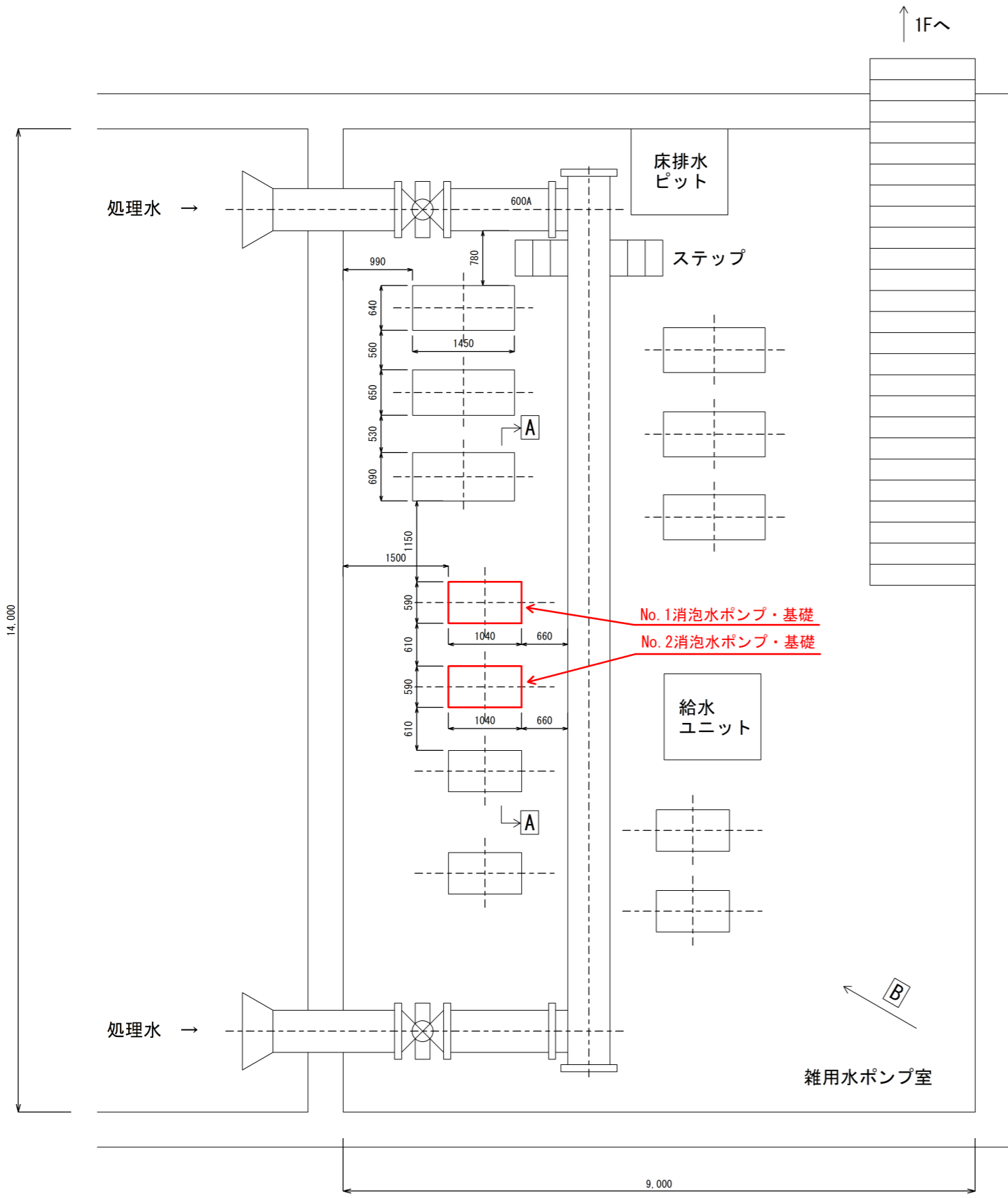
雑用水ポンプ室B1F平面図(1:75)
