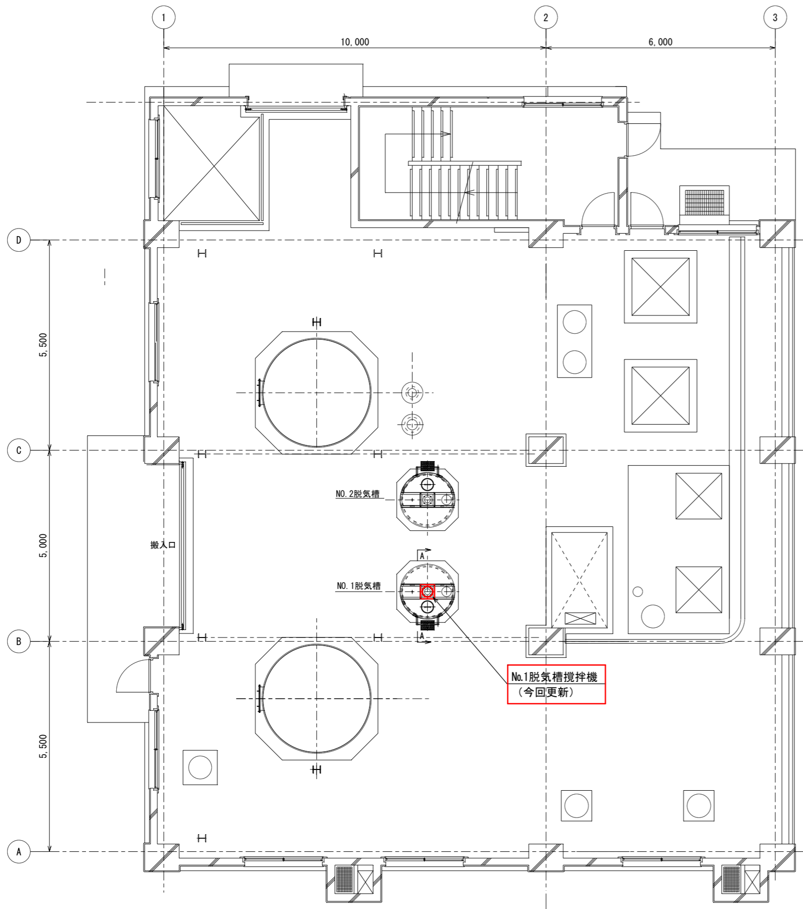
強制濃縮棟1階平面図 S:1/100 (A3)
