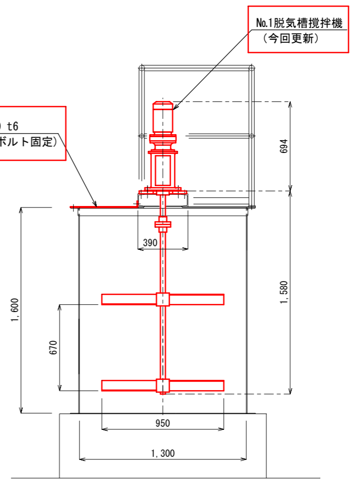
A-A断面 S:1/30 (A3)
