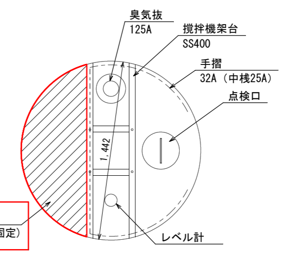
脱気槽蓋平面 S:1/30 (A3)
