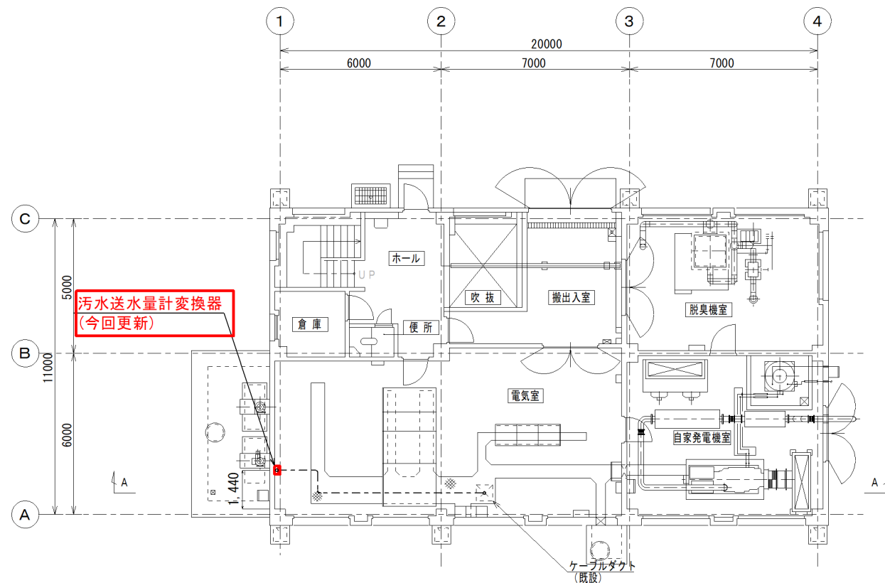
1階 平面図
