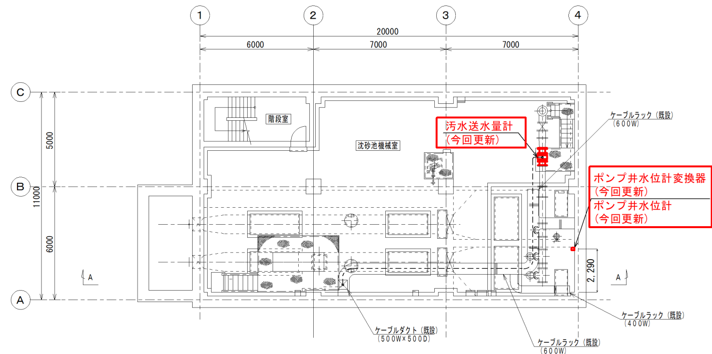
地下1階 平面図
