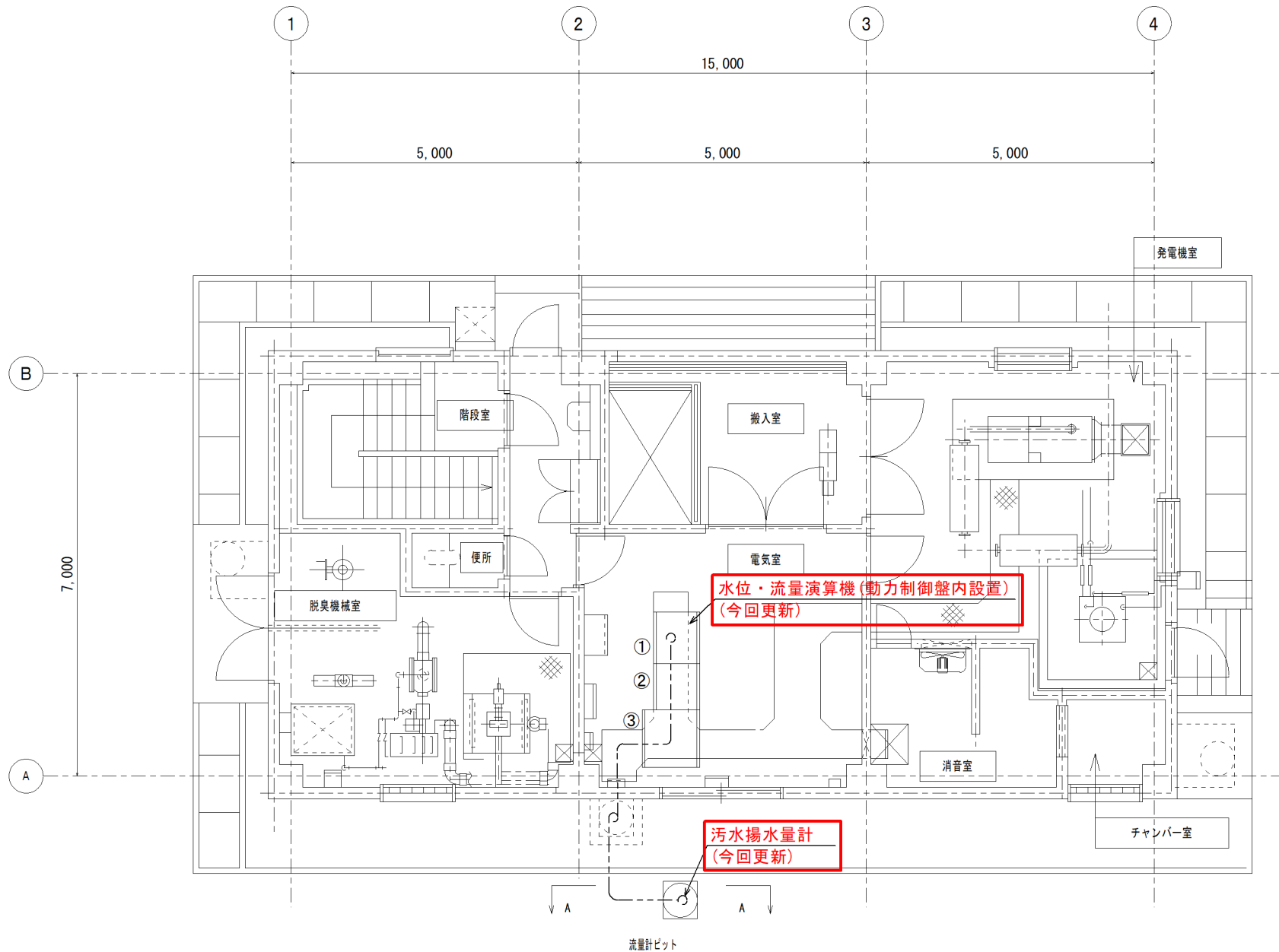
1 階平面図 S:1/100 (A3)
