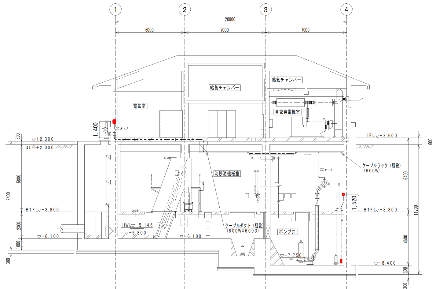
A - A 断面図
