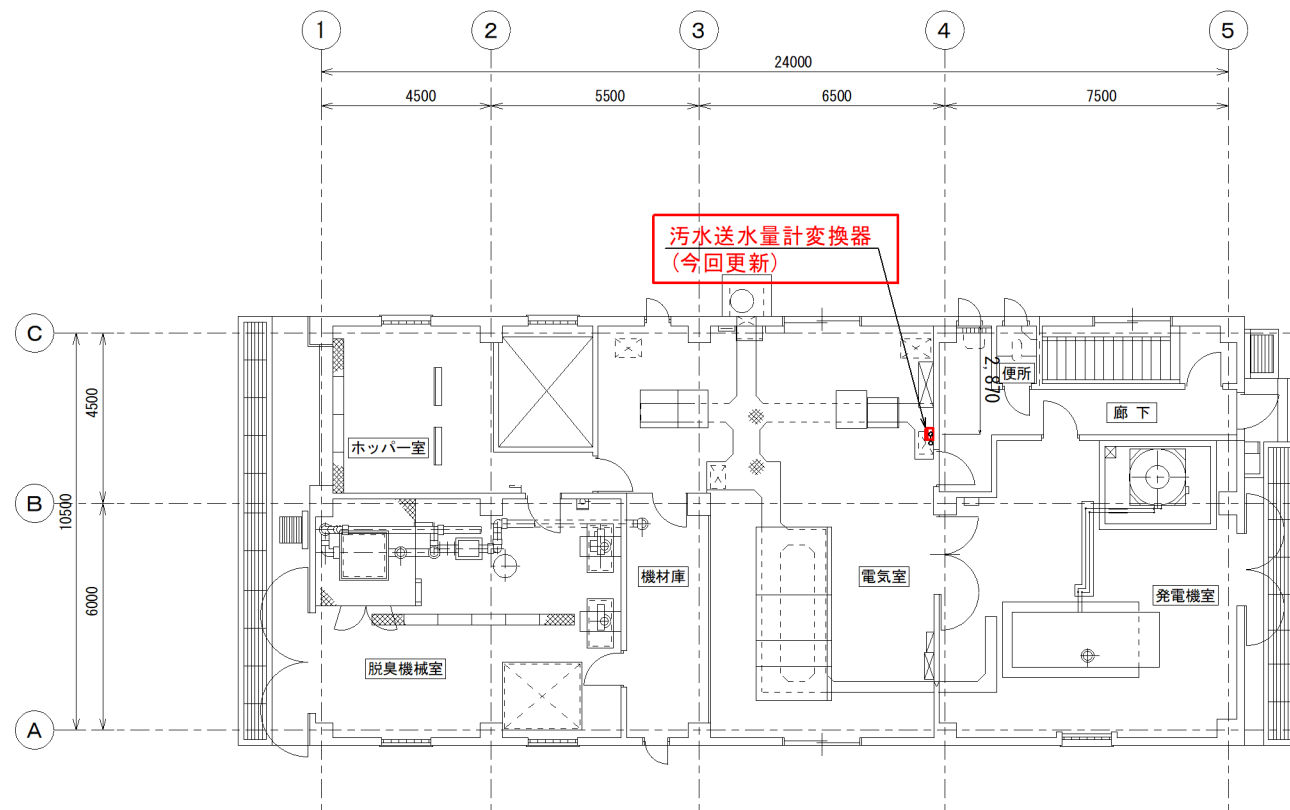
1階 平面図
