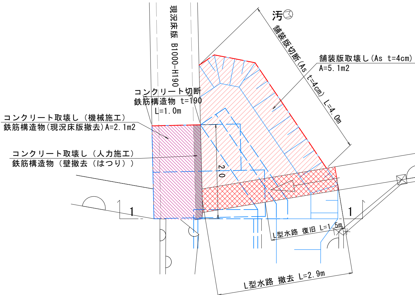
側面図 s=1:50
