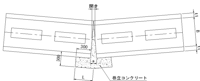
断面図
