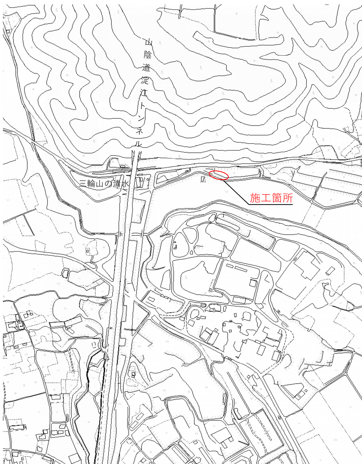
位置図 S = 1 : 5,000
