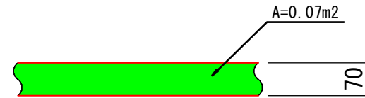
歩車道境界ブロック 断面図
